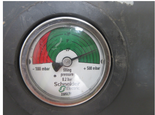
SF6 INDICATOR
